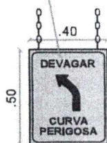
DETALHAMENTO - PLACAS DE ADVERTÊNCIAS ESCALA 1/25
