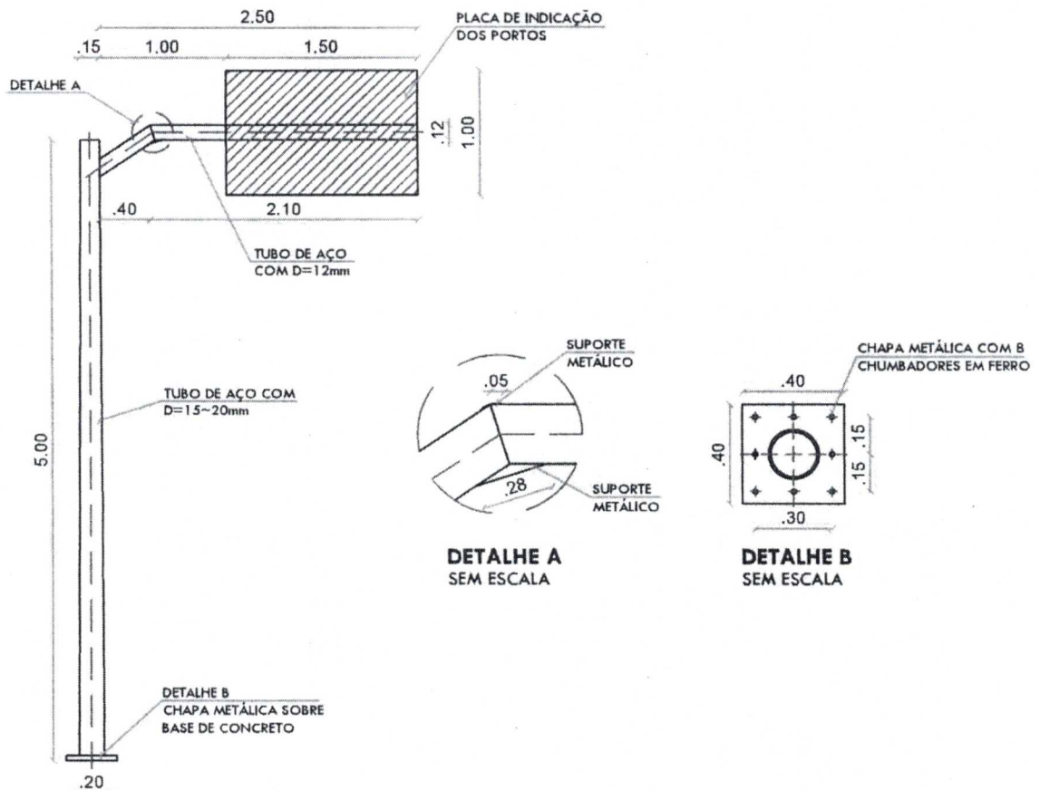
DETALHAMENTO - PORTE COM BRAÇO PROJETADO ESCALA 1/25
