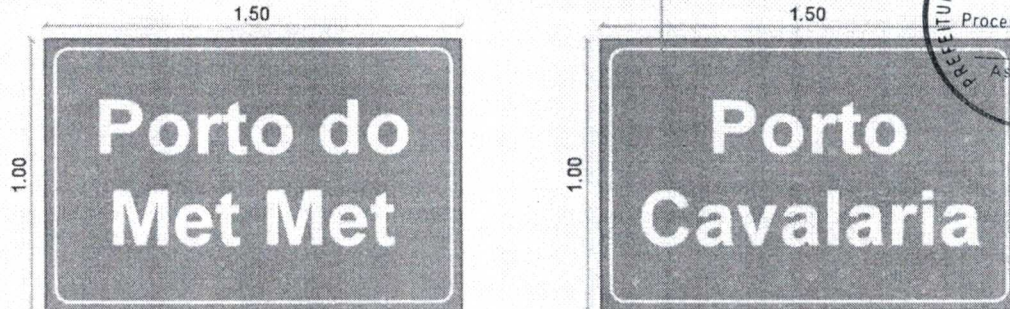
DETALHAMENTO - PLACAS DE INDICAÇÃO DOS PORTOS ESCALA 1/25
