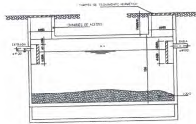
Det. FOSSA SÉPTICA Corte CD-Fossa E.c. 101
