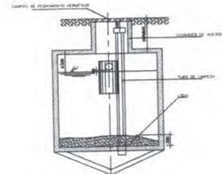
Det. FOSSA SÉPTICA Corte AB-Fossa E.c. 101
