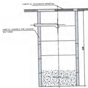
Det. SUMIDOURO Corte LM E.c. 101
