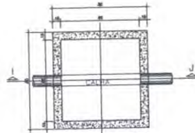
Det. CX. INSPEÇÃO Planta Baixa E.c. 101
