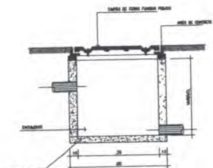
Det. CX. INSPEÇÃO Corte IJ E.c. 101
